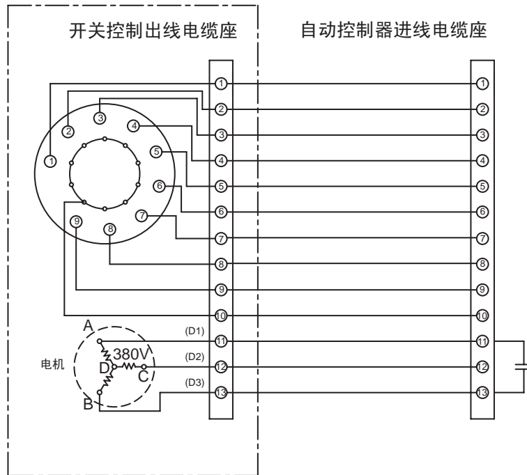
附图13 开关与控制器电气接线图
