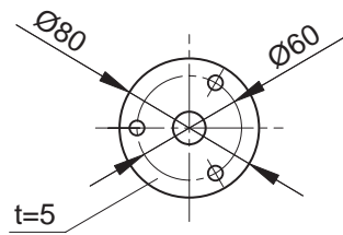
吸湿器安装法兰
